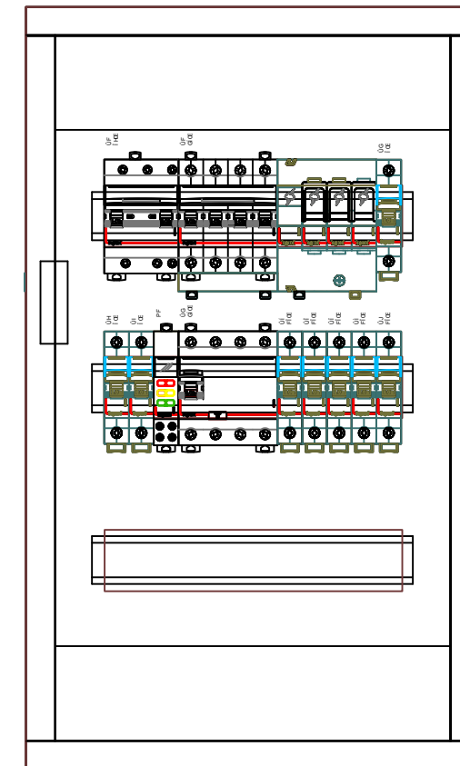
PROJ. ROZDZIELNICA RWN 3x12 P/T IP40
